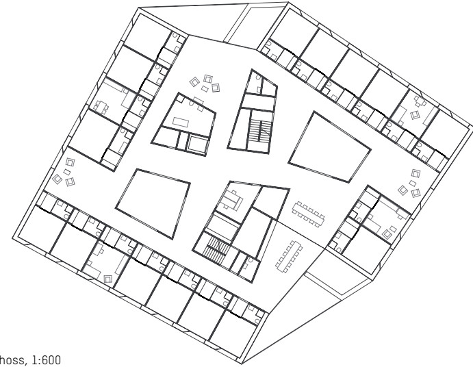
Regelgeschoss, 1:600
